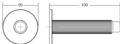
Fijación con tornillo y adhesivo
