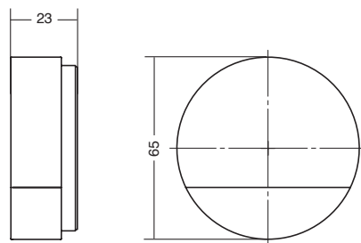
Fijación con adhesivo
