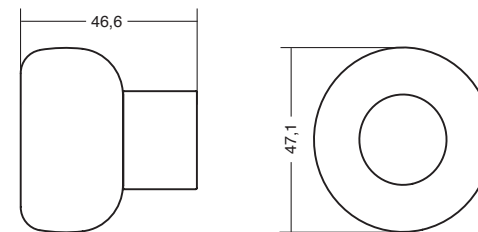
Fijación con tornillo
